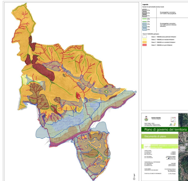
Fattibilità geologica e protezione sismica locale
